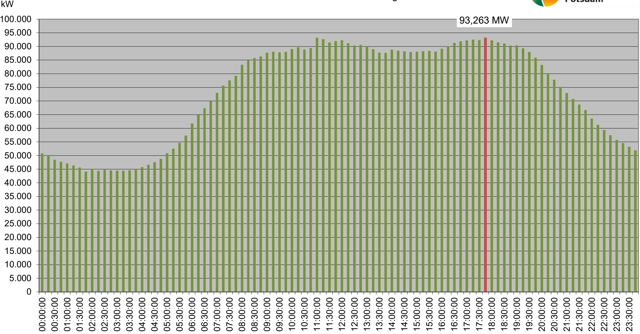
Verlauf der Netzlast HS/MS-Ebene am Höchstlasttag - 05.12.2023
