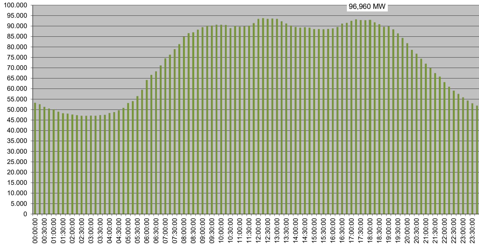
Verlauf der Netzlast HS-Ebene am Höchstlasttag - 11.01.2024
