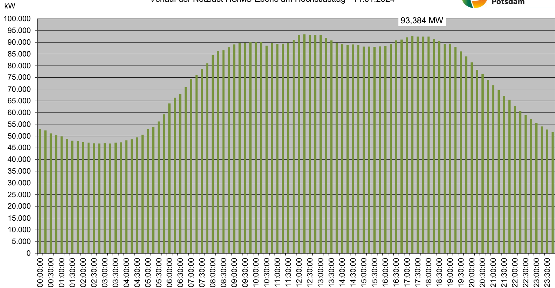
Verlauf der Netzlast HS/MS-Ebene am Höchstlasttag - 11.01.2024
