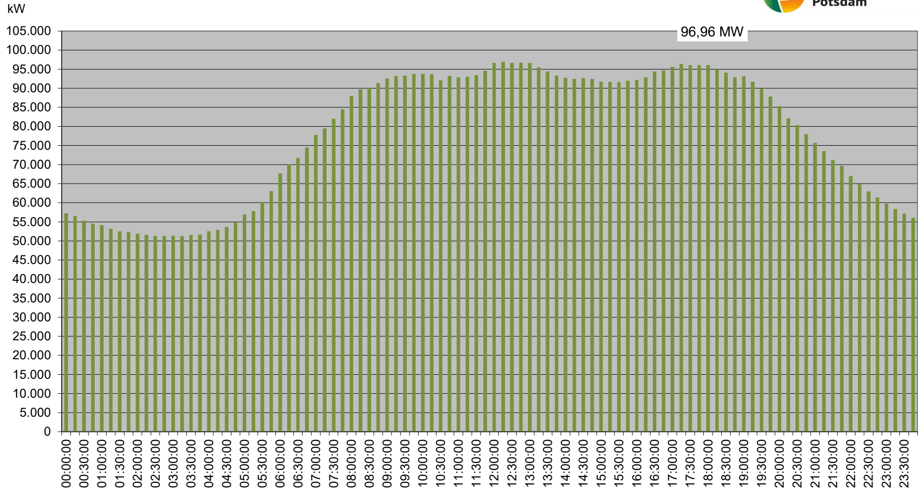
Verlauf der Netzlast MS-Ebene am Höchstlasttag - 11.01.2024
