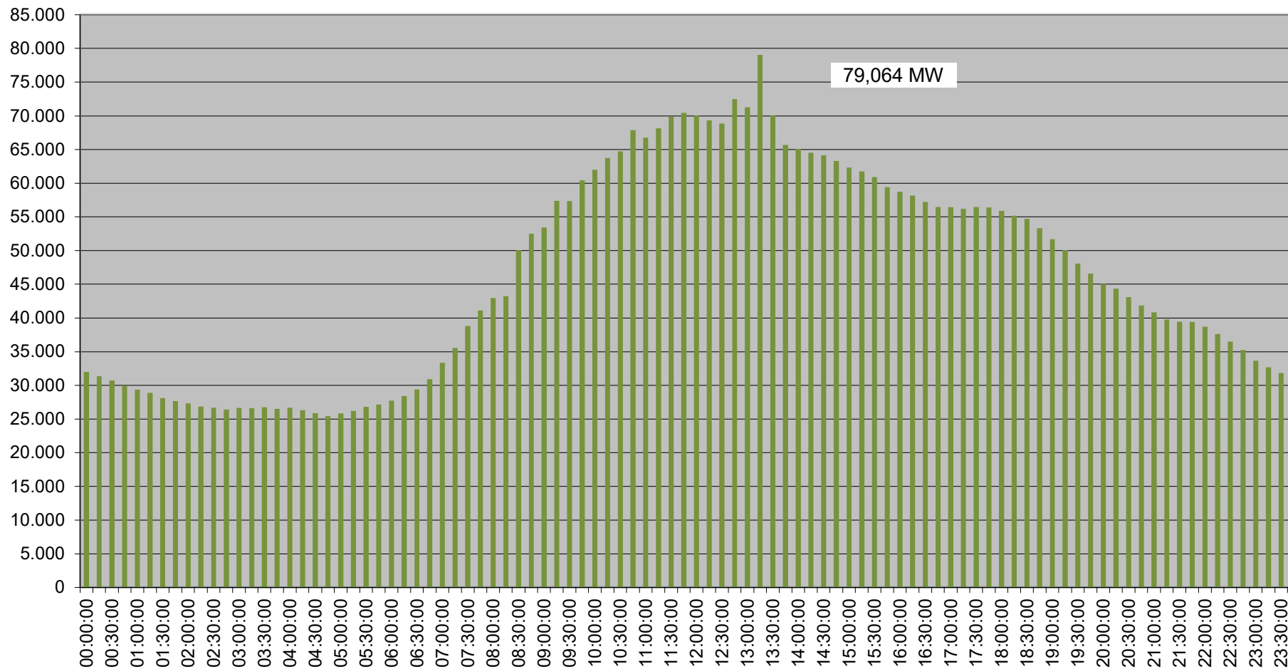
Verlauf der Netzlast MS/NS-Ebene am Höchstlasttag - 09.06..2024
