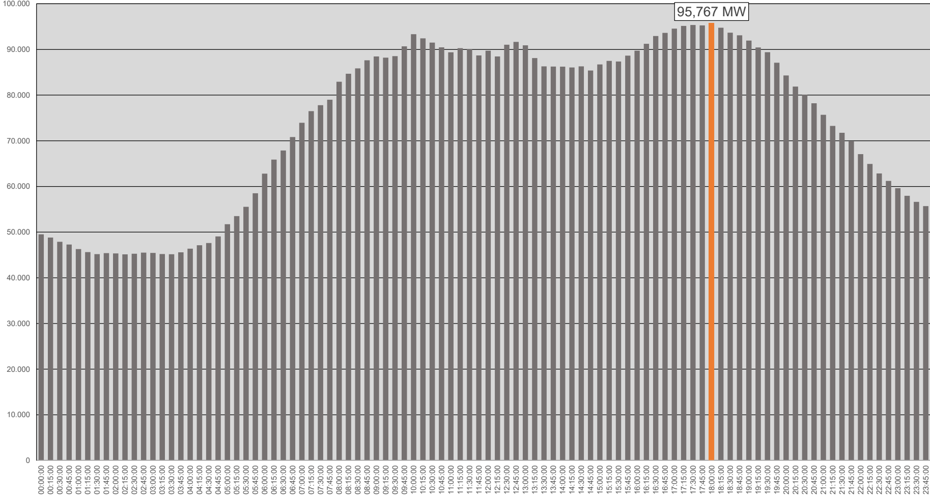
Verlauf der Netzlast HS/MS-Ebene am Höchstlasttag - 24.11.2025
