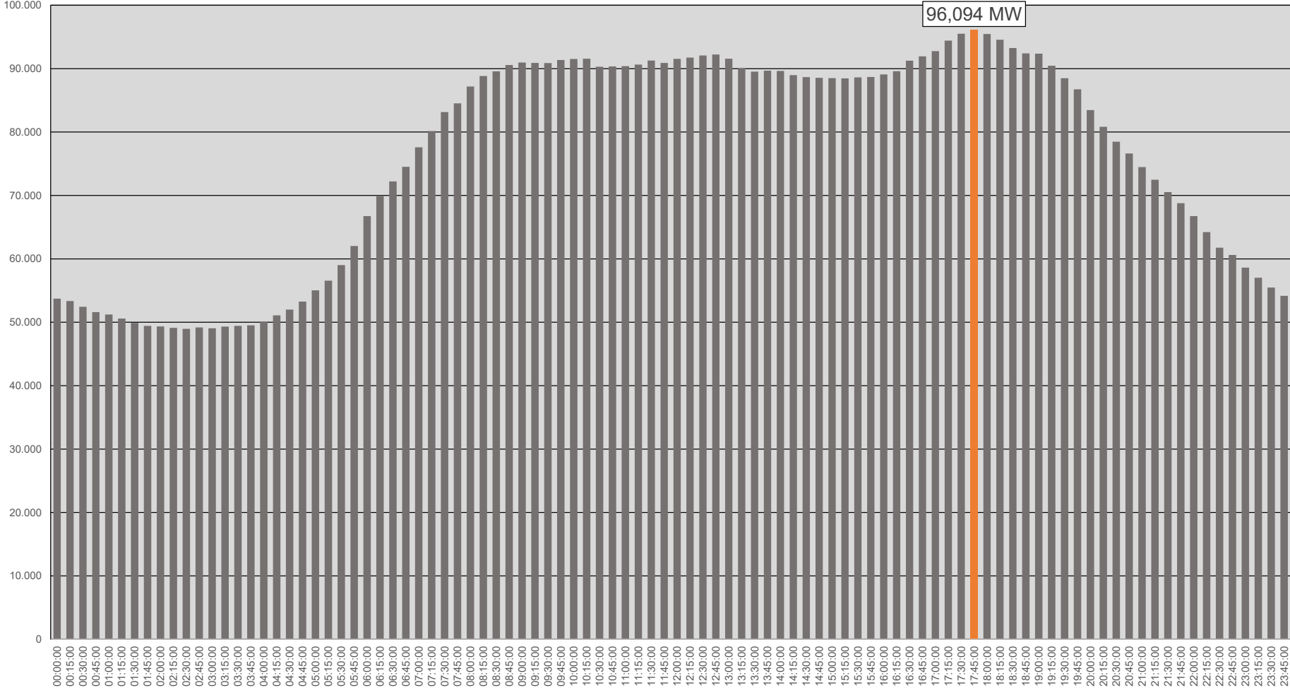
Verlauf der Netzlast MS-Ebene am Höchstlasttag - 14.01.2025
