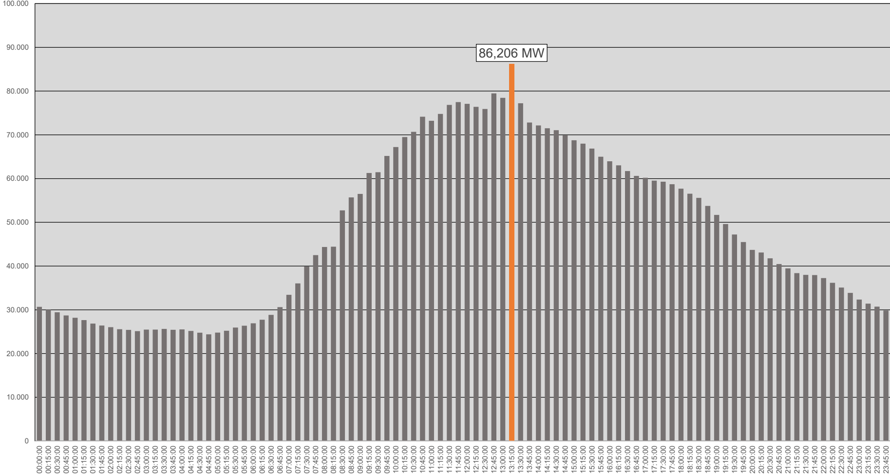
Verlauf der Netzlast NS-Ebene am Höchstlasttag - 10.06.2025
